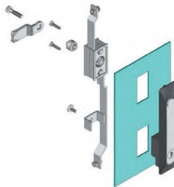
Монтажное отверстие
