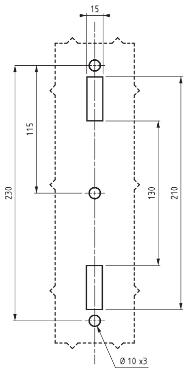
Монтажное отверстие
