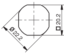
Монтажное отверстие
