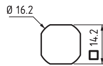
Монтажное отверстие
